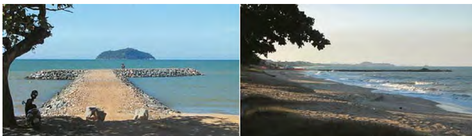
Figura 10 – Imagem mostrando diques construídos em 2011/2012, obra que faz parte, junto com novo aterro hidráulico, do atual projeto de recuperação da praia de Piçarras
