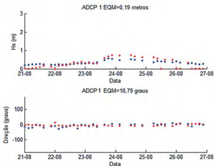
Figura 3 – Calibração do modelo Oluca para enseada de Itapocoró
