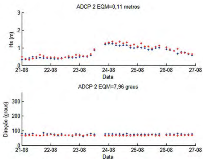
Figura 4 – Calibração do modelo Oluca para enseada de Itapocoró
