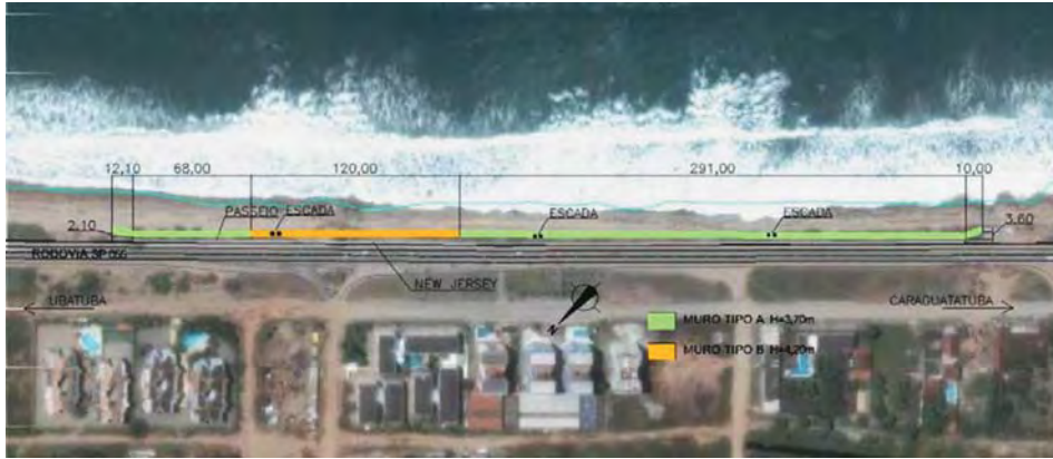
Figura 4 – Forma em planta do muro de pedra argamassada localizado na zona de erosão na praia de Massaguaçu
