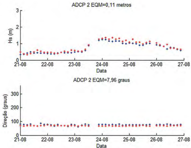
Figura 4 – Calibração do modelo Oluca para enseada de Itapocoróri
