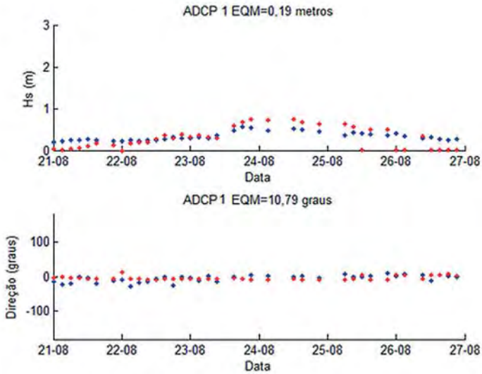
Figura 3 – Calibração do modelo Oluca para enseada de Itapocoróri
